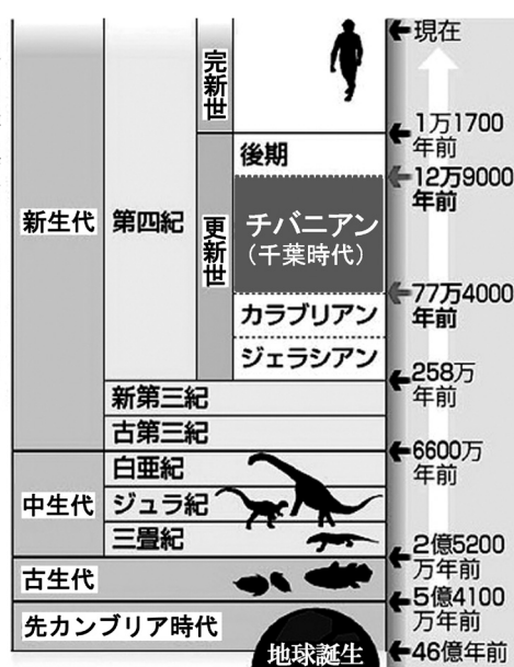
主な地質時代(国際年代層序表)
